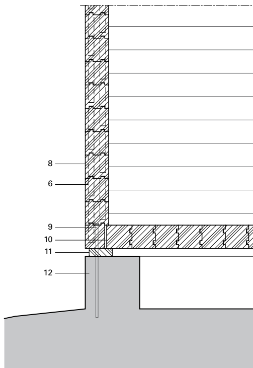
Fassadenschnitt, M 1:20
