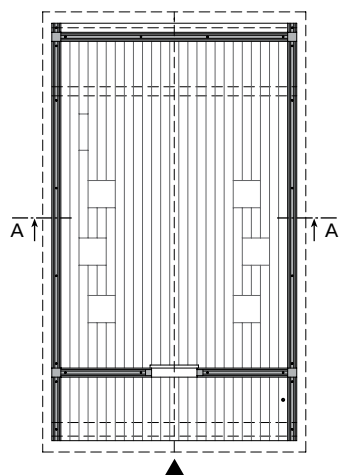
Grundriss, M 1 : 100
