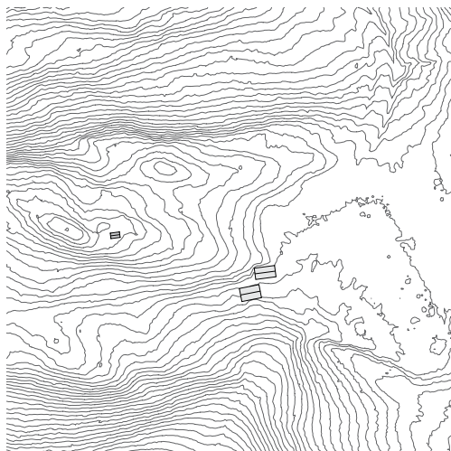
Lageplan, M 1:4000
